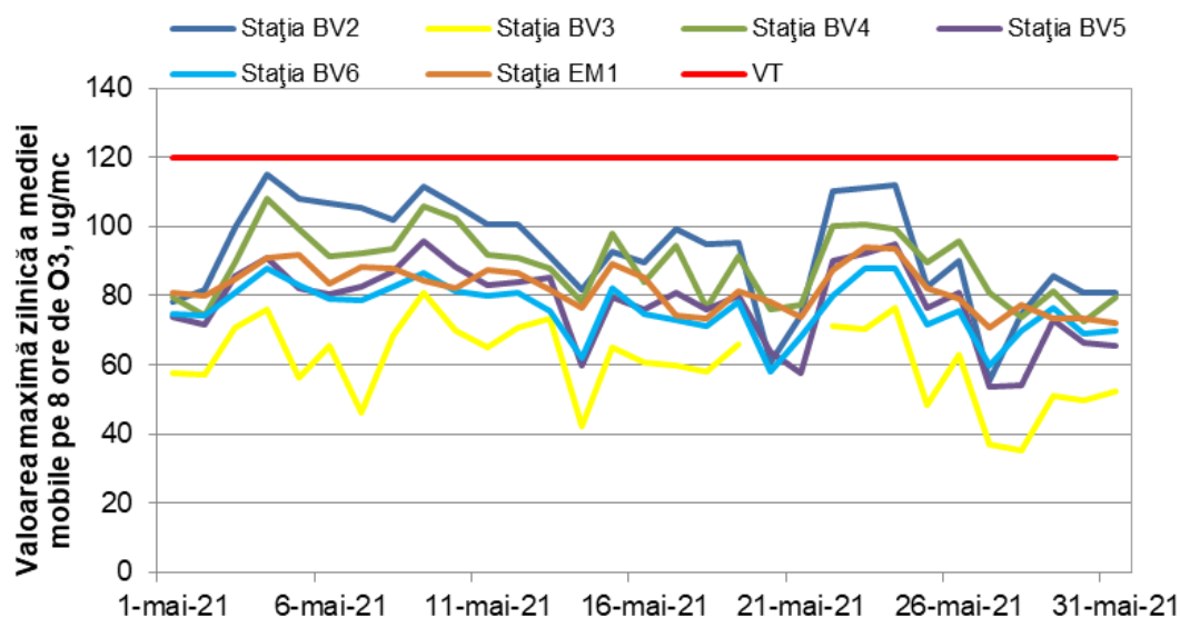
Figura 1.1.2.3.1. Evoluția maximelor zilnice ale mediilor mobile pe 8 ore de \text{O}_3 în luna mai
