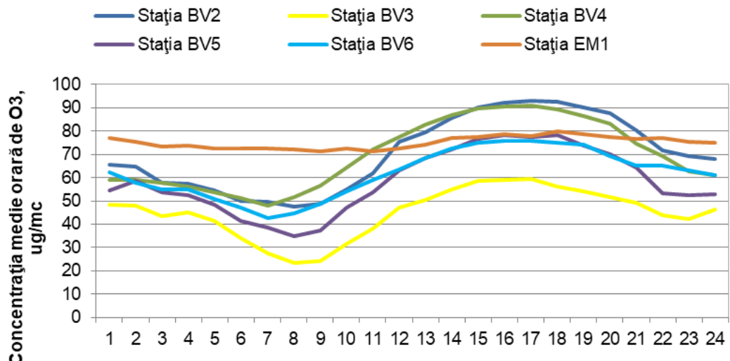
Figura 1.1.2.3.2. Ciclul zilnic al ozonului
