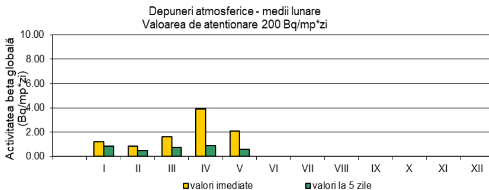
Fig. 1.3.4. Activitatea beta globală pentru depuneri atmosferice
