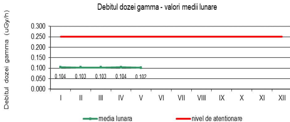
Fig. 1.3.3. Debitul dozei gamma în aer
