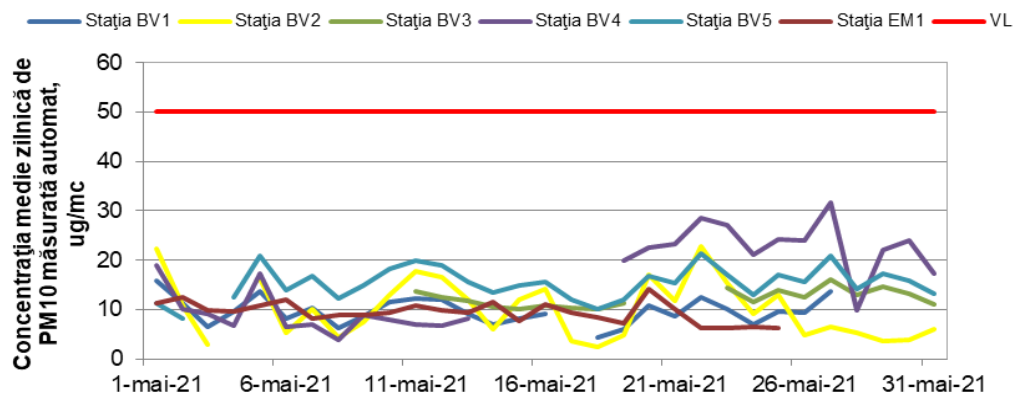
Figura 1.1.2.4.1. Evoluția mediilor zilnice de PM 10 în luna mai
