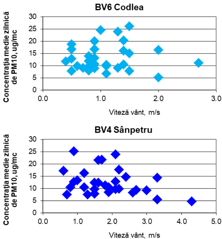
Figura 1.1.2.4.2. Evoluția mediilor zilnice de PM 10 în funcție de viteza vântului
