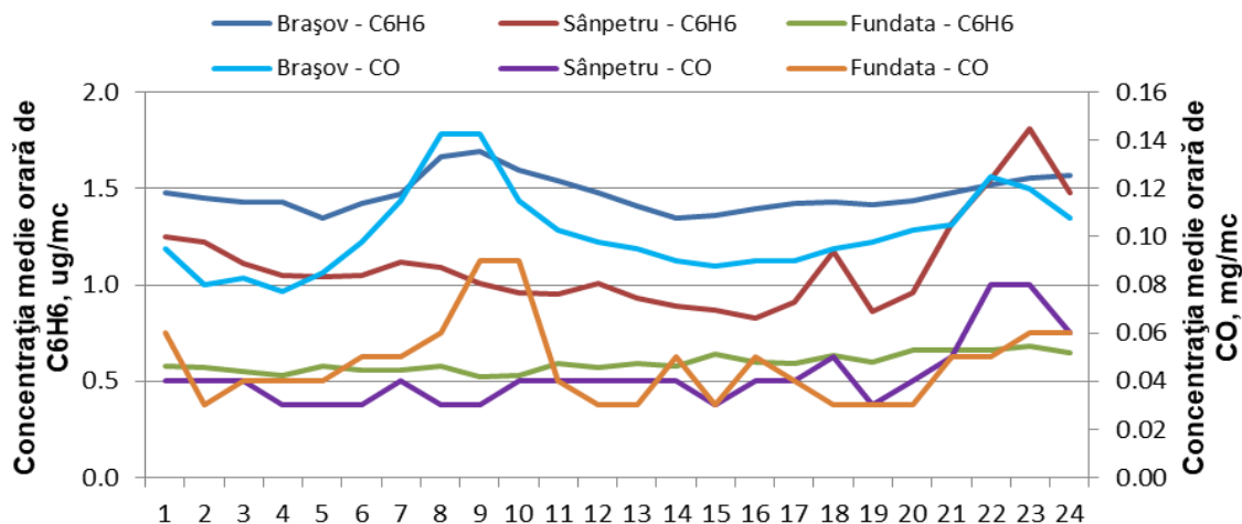
Figura 1.1.2.6.2: Ciclu zilnic al CO și benzenului în Brașov
