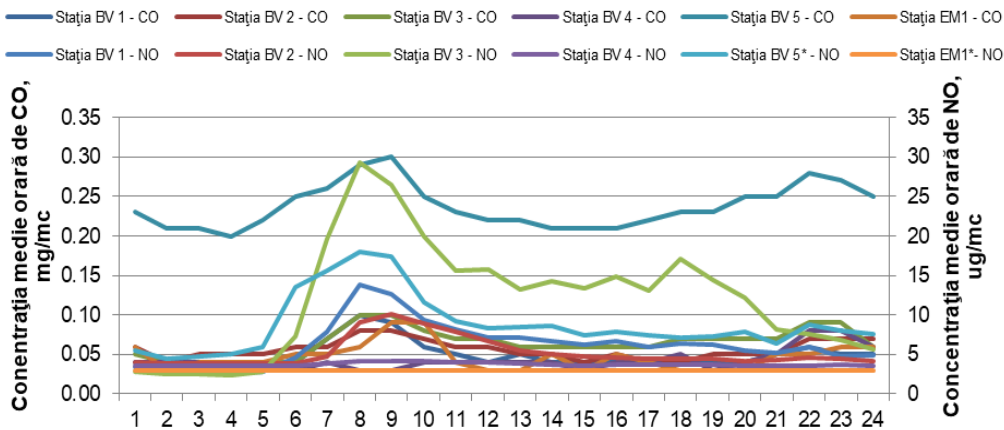
Figura 1.1.2.2.4. Ciclul zilnic al \text{NO} și \text{CO}
