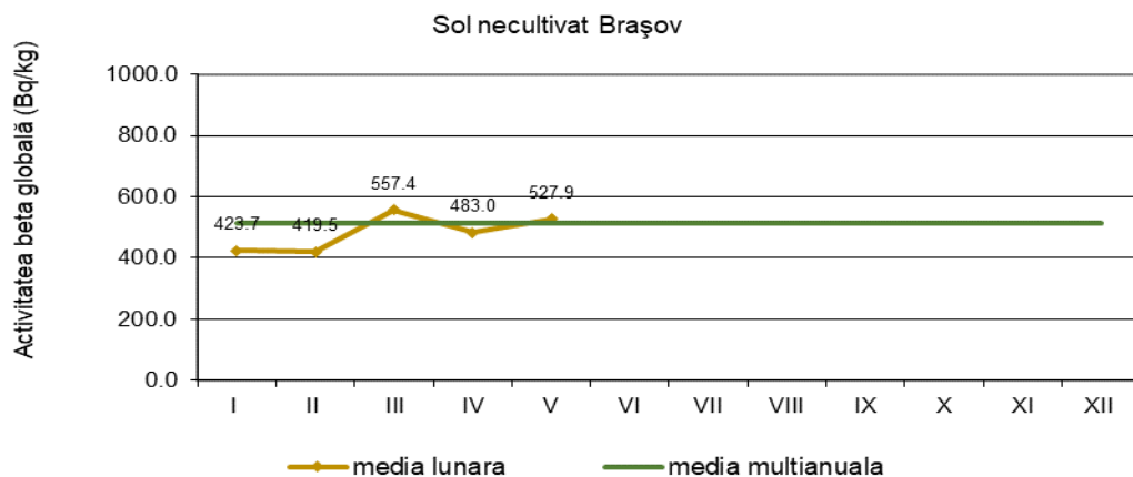
Fig. 1.3.8. Activitatea beta globală la 5 zile pentru solul necultivat
