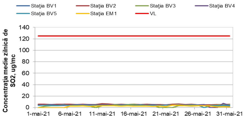
Figura 1.1.2.1.1. Evoluția mediilor zilnice de SO 2 în luna mai
